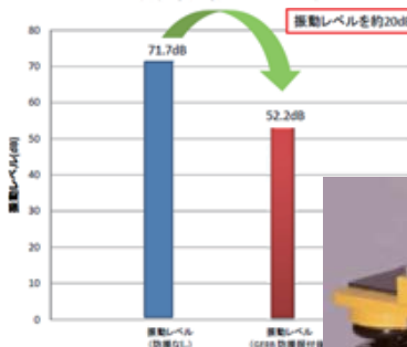
GERB防振装置据付け前後の振動レベル
